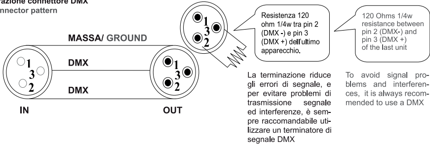
Configurazione connettore DMX DMX connector pattern
