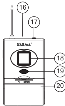
Microfono bodypack
