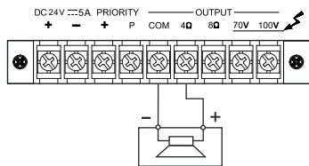
Connessione Speakers a 4 Ohms
