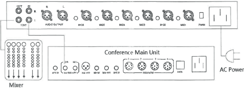
2) Schema di collegamento con conference system.
