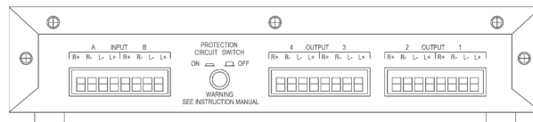
Connettori posteriori
