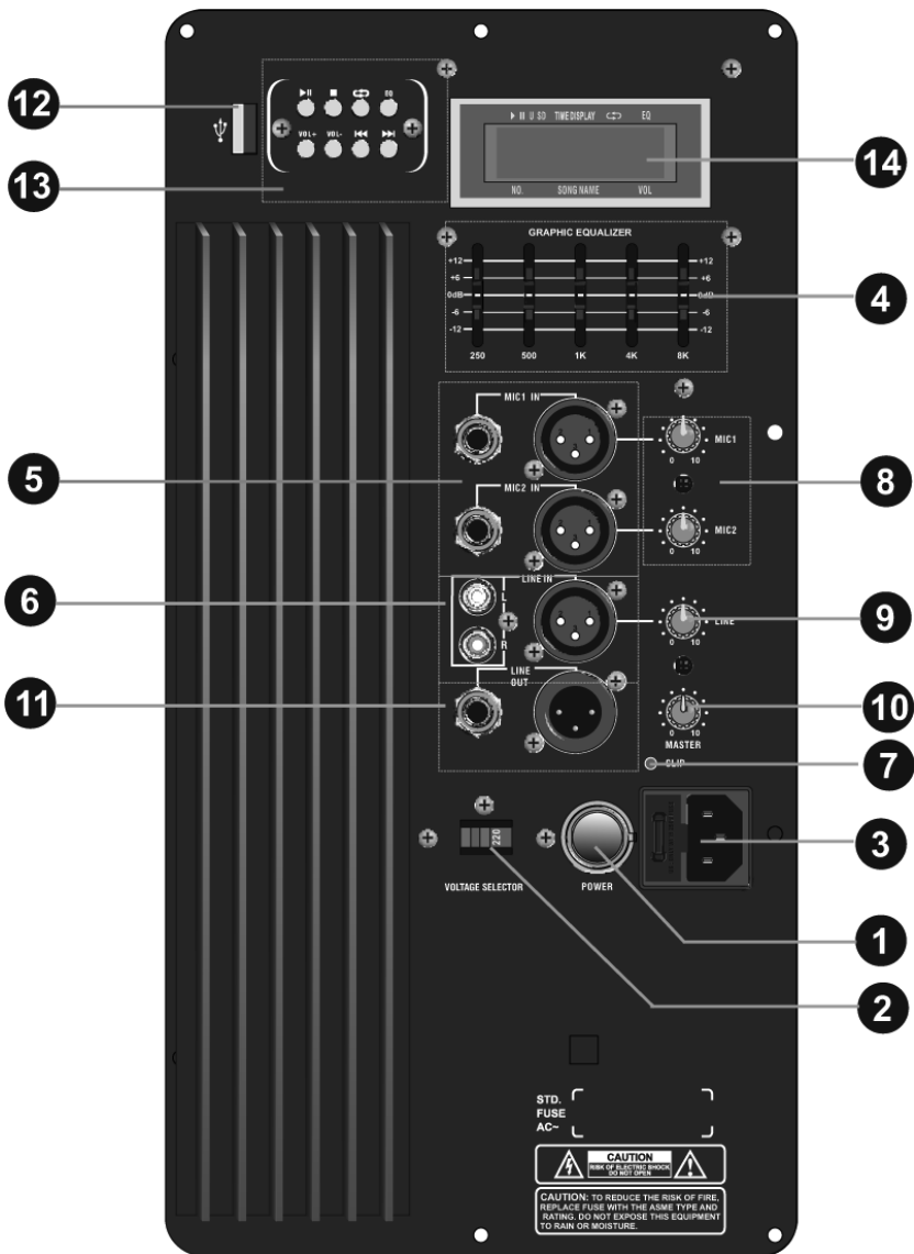
Pannello posteriore
