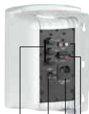
Pannello posteriore Serie BS 59BA e BS 59WA attivo
