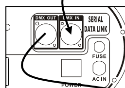
Illustrazione del pannello di ingress/uscita di un effetto luce
